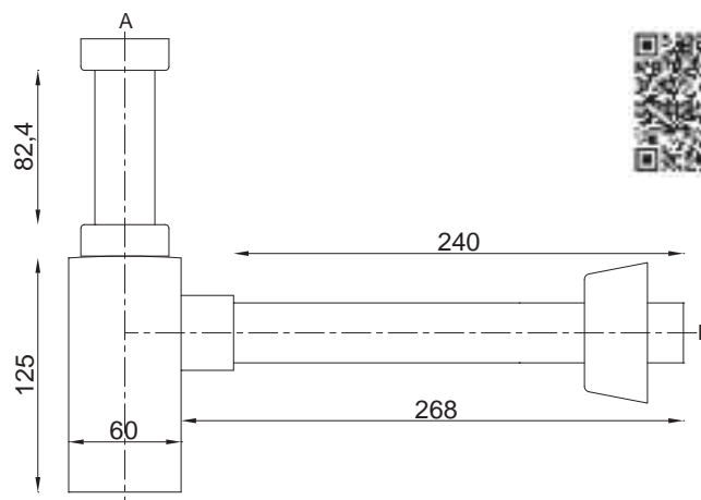
Sifone minimalista QUADRO da 1"1/4 per lavabo in ABS
