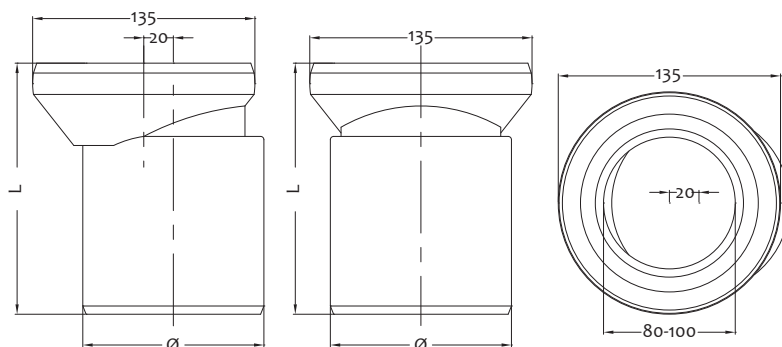
Manicotto rigido WC eccentrico Ø110
