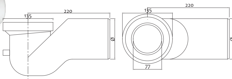
Curva tecnica in materiale plastico
