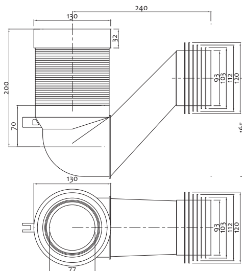
Curva tecnica disassata per ristrutturazione accorciabile Cutable offset WC bend for rebuilding
