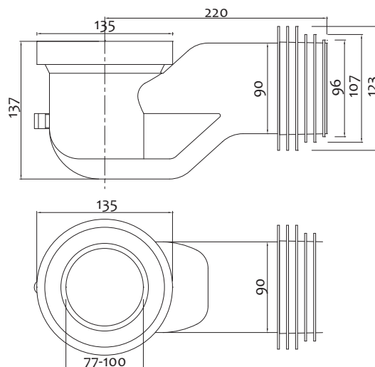
Curva sottovaso guarnizione alettata universale WC bend with finned universal gasket
