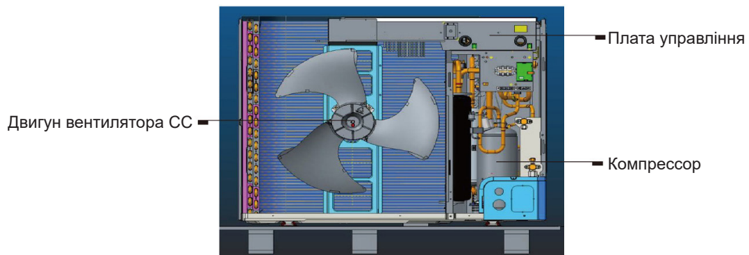
Вид зсередини
