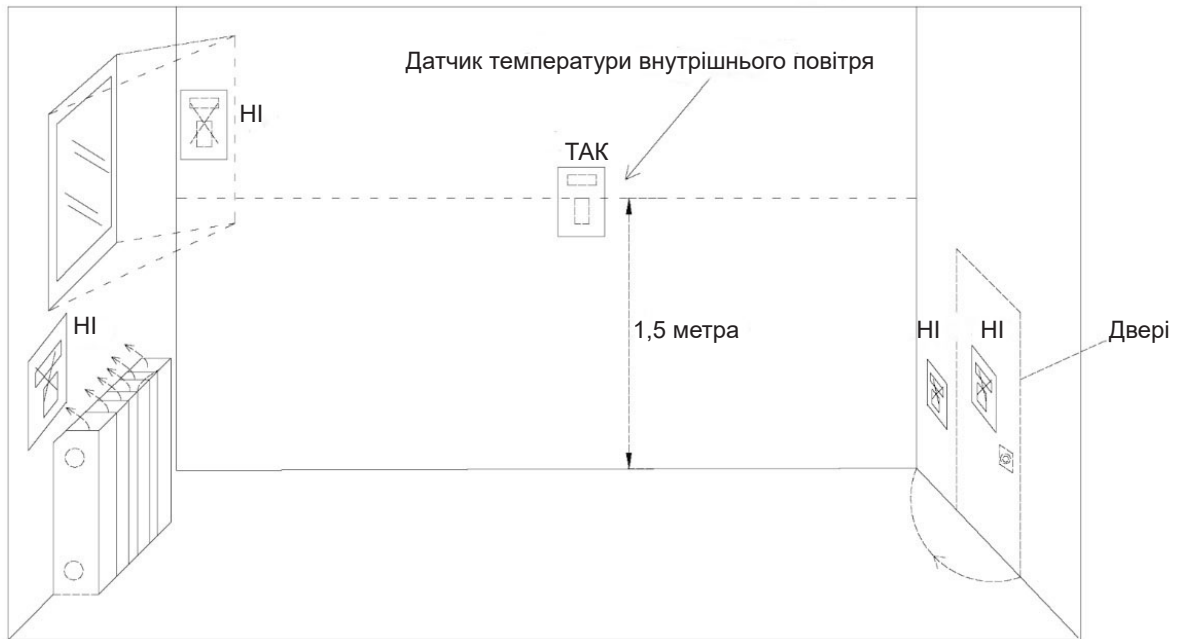
Фронтальний вид
